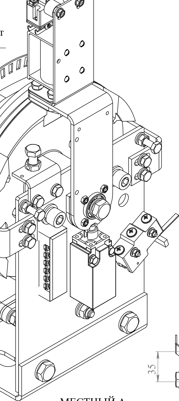
МЕСТНЫЙ А МАСШТАБ 1 : 1
